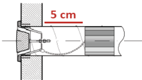
Asennus seinässä olevaan kanavaan
