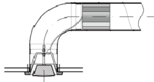
Asennus katossa olevaan kanavaan
